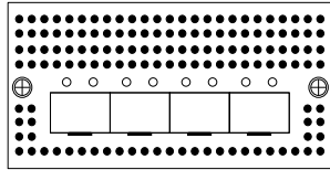
LANCOM UF Extension Module 4× 1G SFP (UF-500 / UF-9XX)
